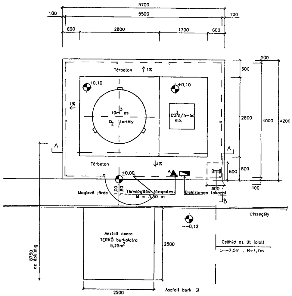
ALAPRAJZ
