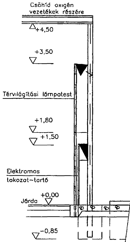
B NÉZET
