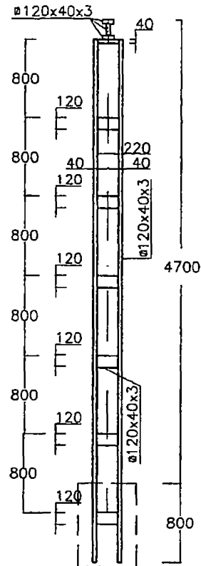
OSZLOP NÉZETI RAJZA
