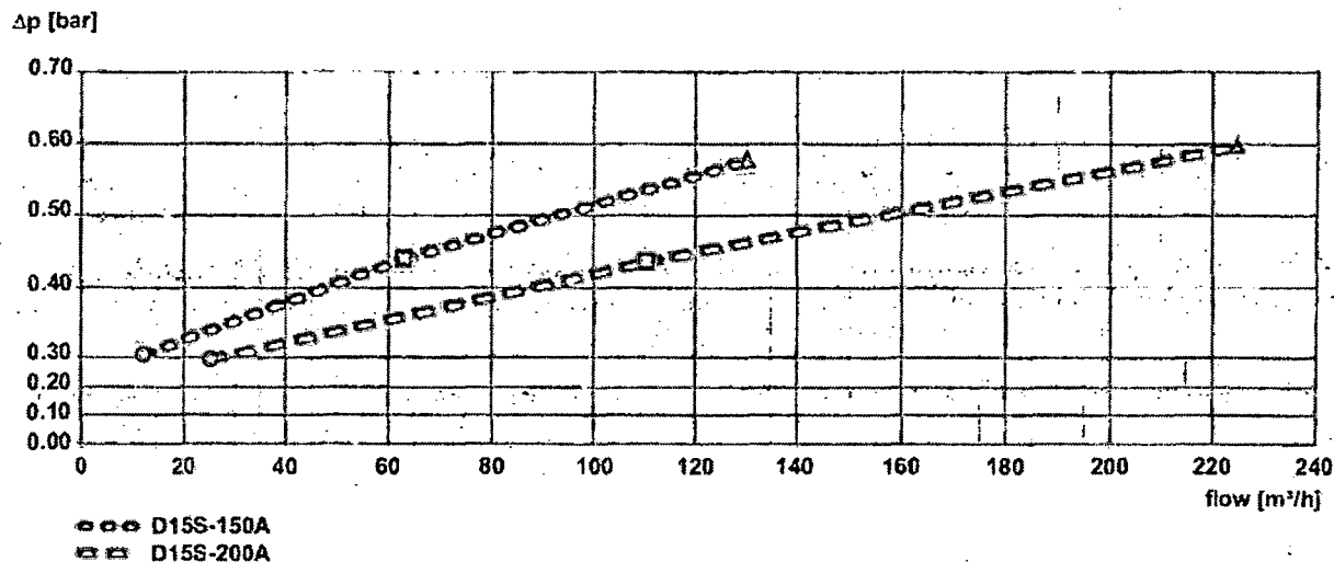
3. ábra Nyomásesés a szelepből az átfolyás és az alkalmazott csatlakozó méret függvényében (Méretek: 150-200) Nyomásbeállítás: P1: 8 bar, P2: 3 bar
