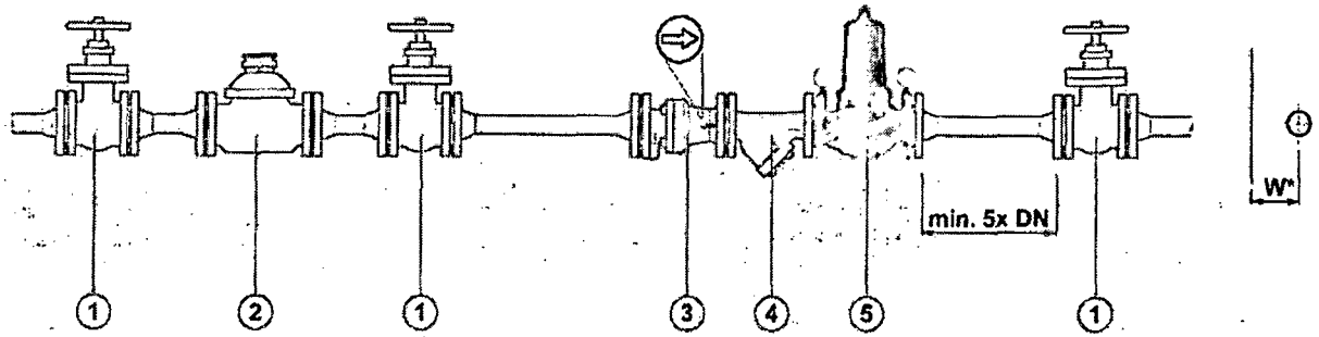
1. ábra Példa a nyomásszabályozó szelep szokásos beépítésére
