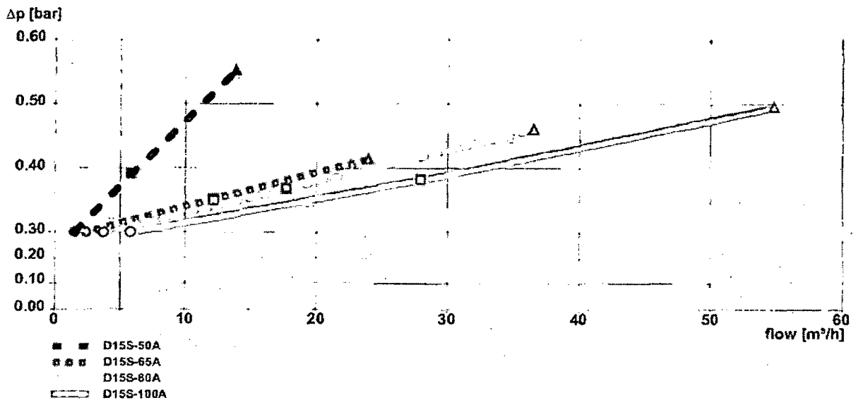
2. ábra Nyomáscsökkentés a szelepekben az átfolyás és az alkalmazott csatlakozó méret függvényében (Méret: 50-100) Nyomásbeállítás: P1: 8 bar, P2: 3 bar
