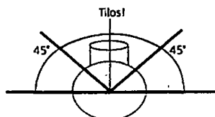
47. ábra KGEA 45°-os ívdomok beépítési korlátozása
