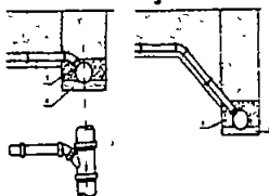
47. ábra KGEA 45°-os ívdomok beépítési korlátozása
