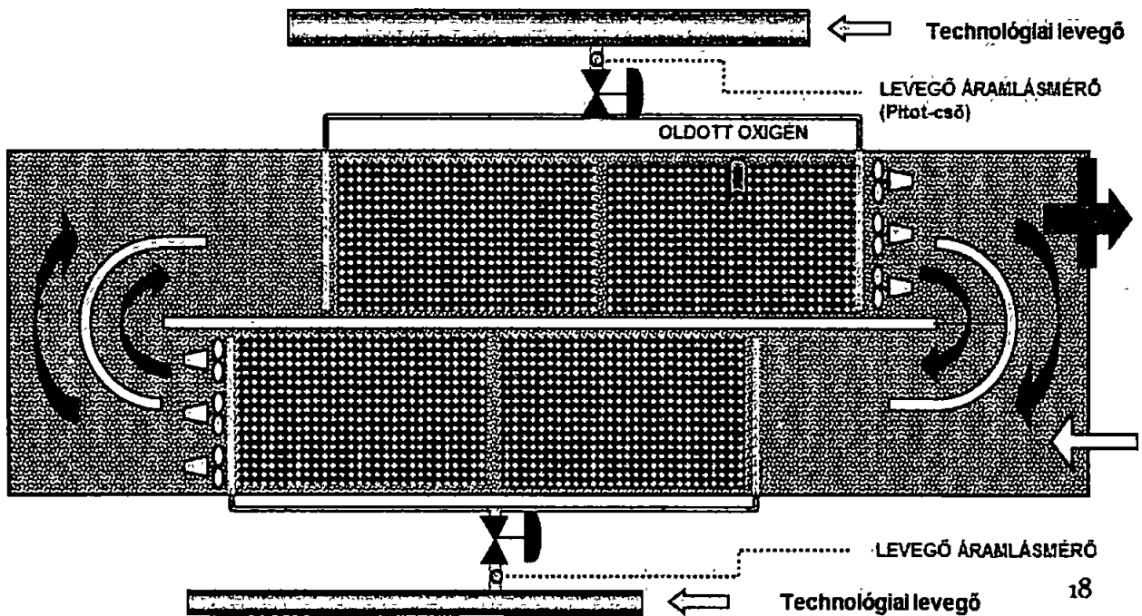
2. ábra: A levegőtető rendszer sematikus elrendezése és szerelvényei
